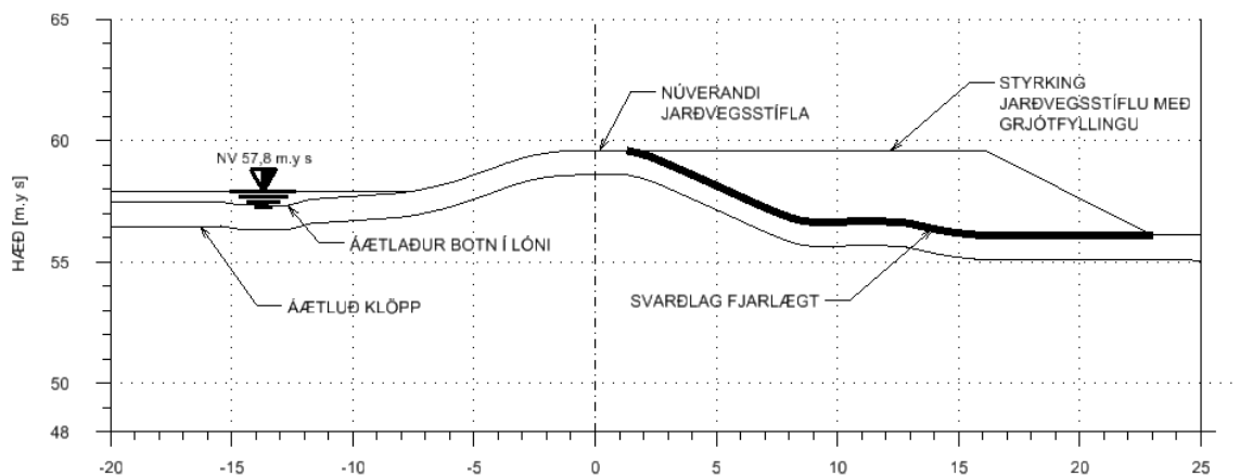
Mynd 4: Snið í núverandi stíflu og styrkingu sem koma skal fyrir.
