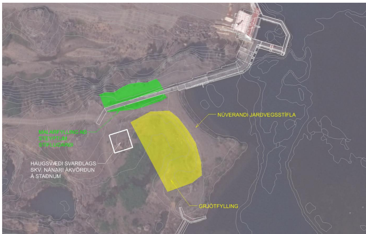
Mynd 2: Yfirlitsmynd af núverandi stíflu með nýrri styrktarfyllingu loftmegin
