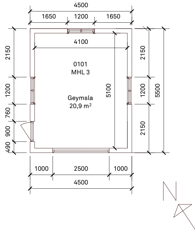
Grunnmynd 1. Hæð 1:100
