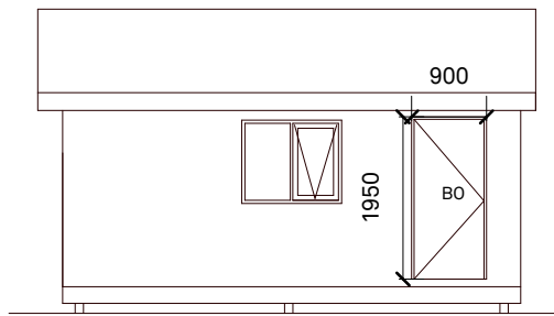
Útlit: Vestur 1:100
