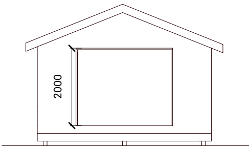
Útlit: Norður 1:100
