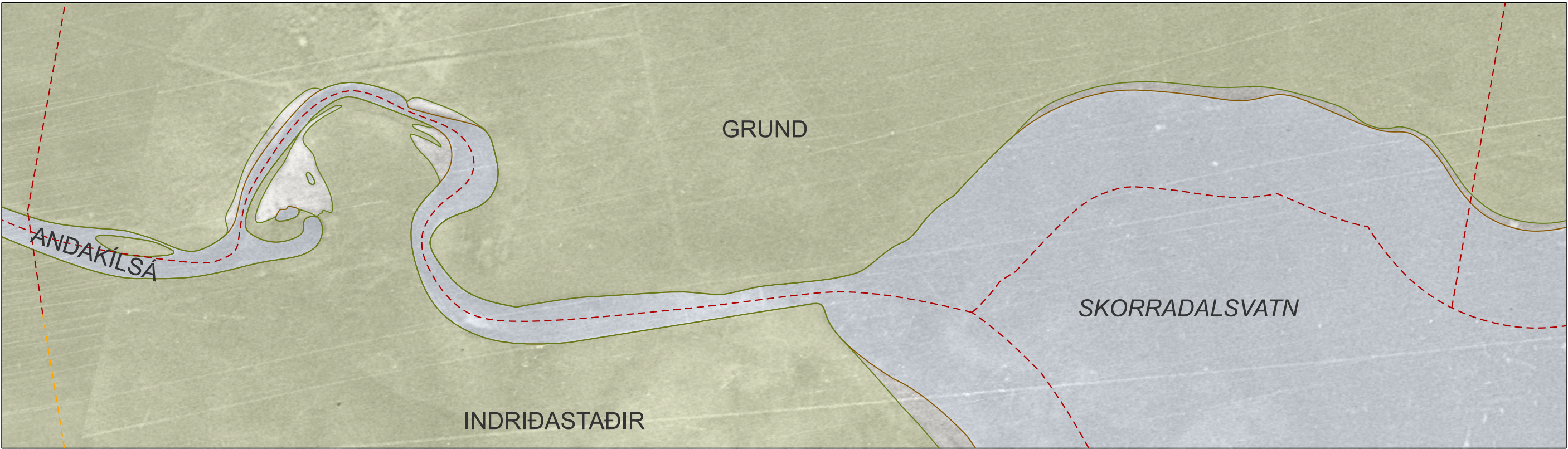
STRAND- OG GRÓÐURLÍNA ÁRIÐ 1945
