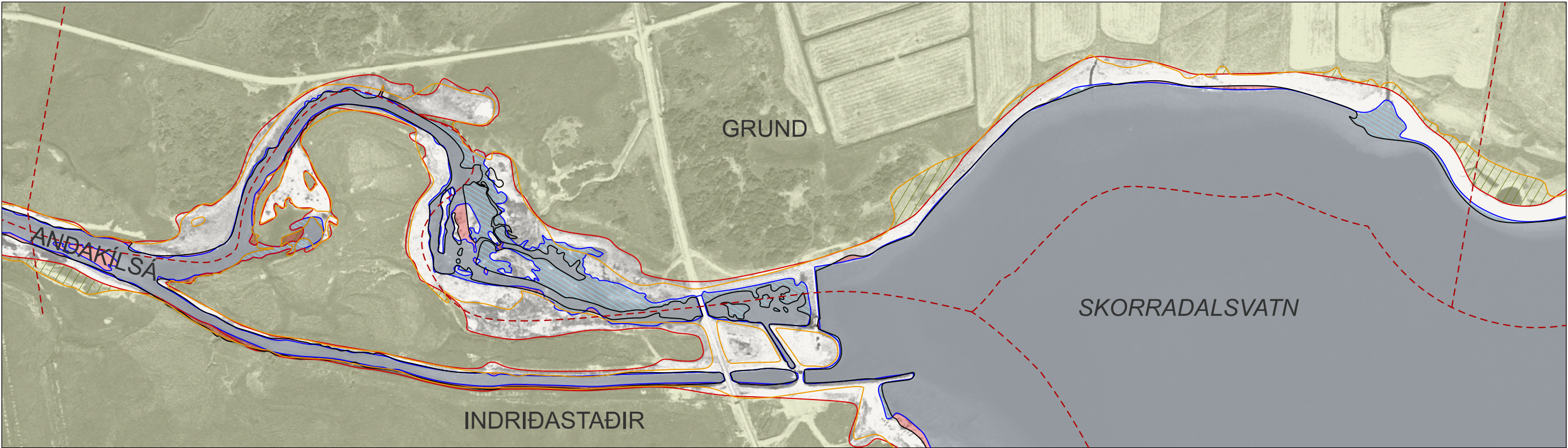
BREYTING Á STRAND- OG GRÓÐURLÍNU FRÁ 1994 OG 2005
