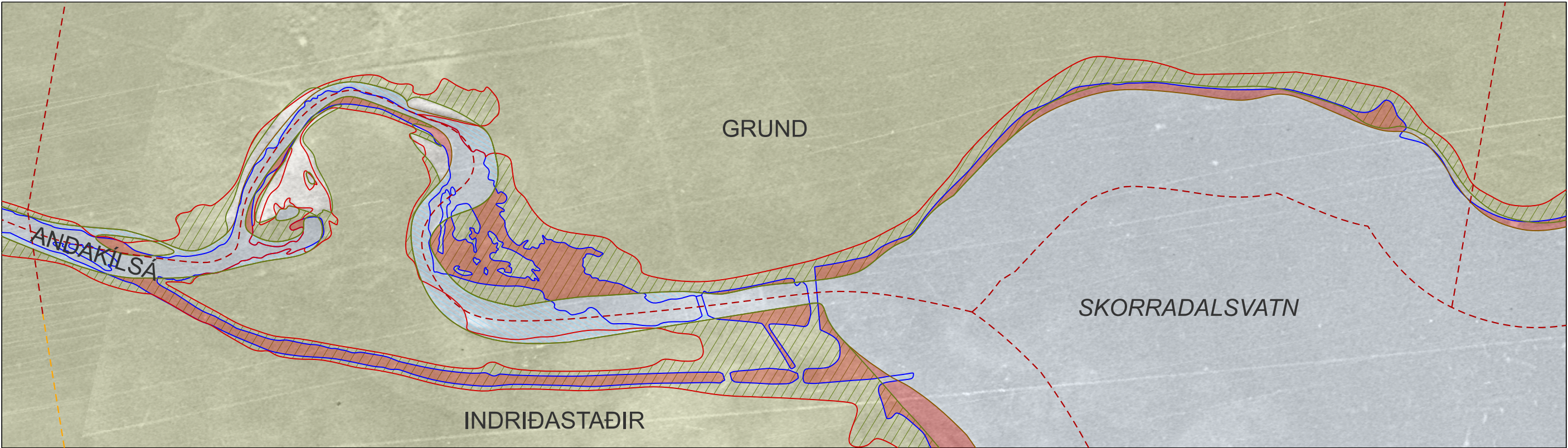
BREYTING Á STRAND- OG GRÓÐURLÍNU FRÁ 1945 OG 1994
