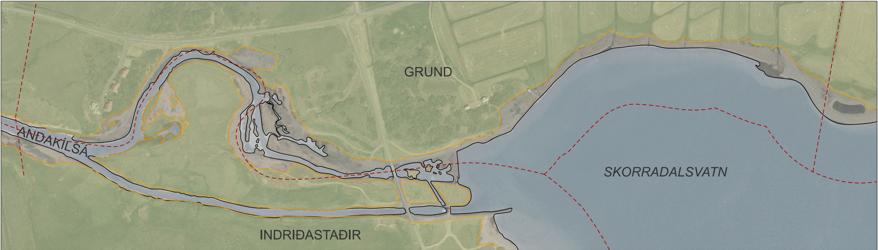
STRAND- OG GRÓÐURLÍNA ÁRIÐ 2005
