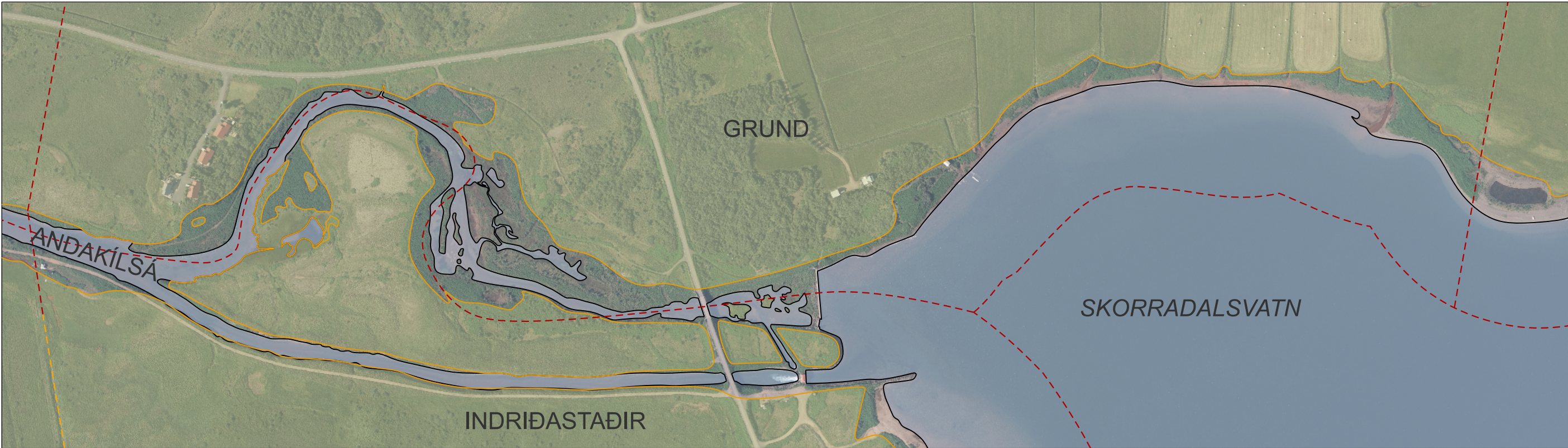
STRAND- OG GRÓÐURLÍNA ÁRIÐ 2024
