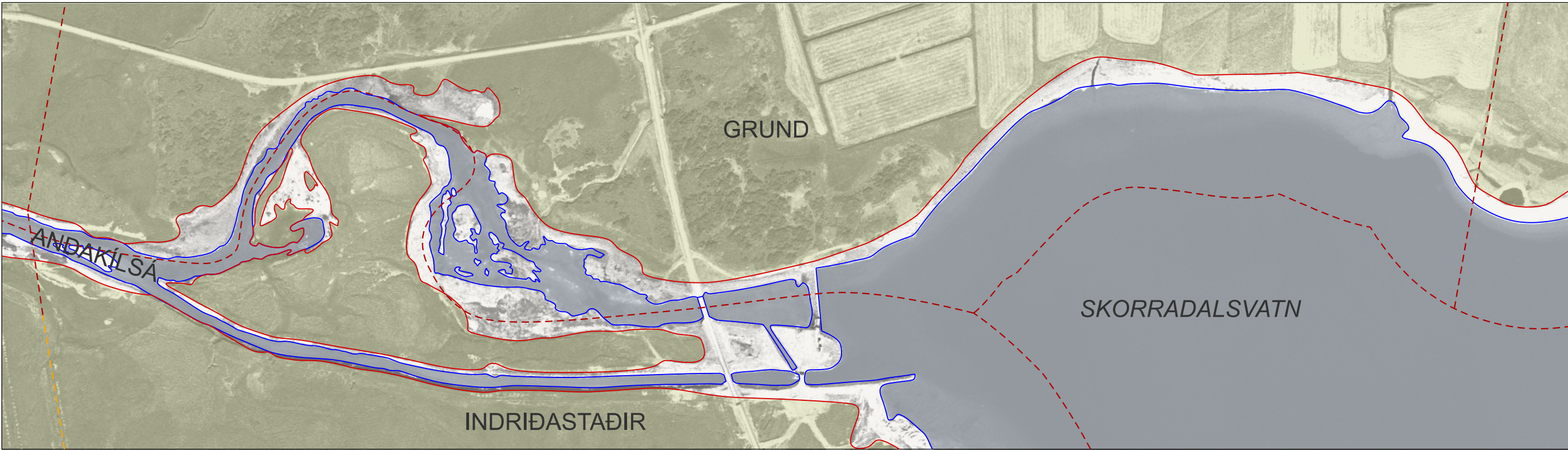
STRAND- OG GRÓÐURLÍNA ÁRIÐ 1994
