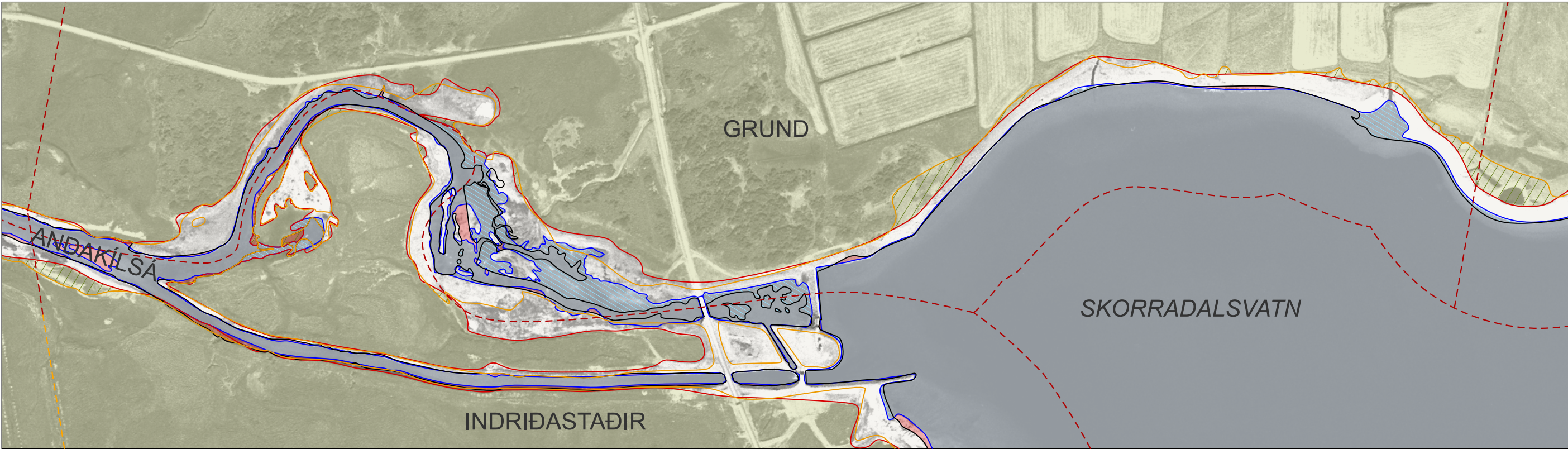
BREYTING Á STRAND- OG GRÓÐURLÍNU FRÁ 1994 OG 2024
